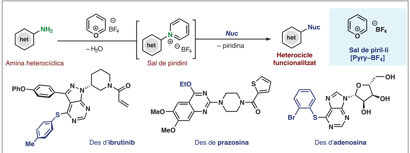
FIGURA 2. Activació d'amines heterocíciques mitjançant una sal de piril·li. Elaboració pròpia.
