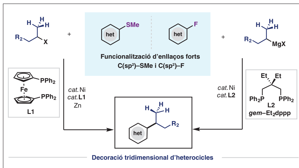
FIGURA 1. Decoració de cicles heteroaromàtics a partir de la catàlisi de níquel. Elaboració pròpia.
